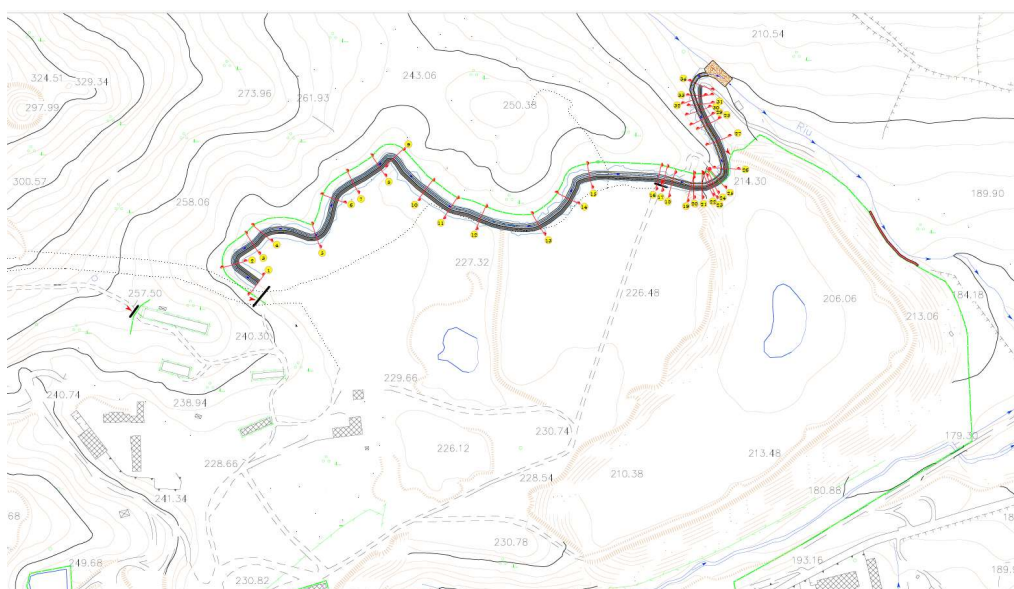
Planimetria del canale di guardia da realizzare
